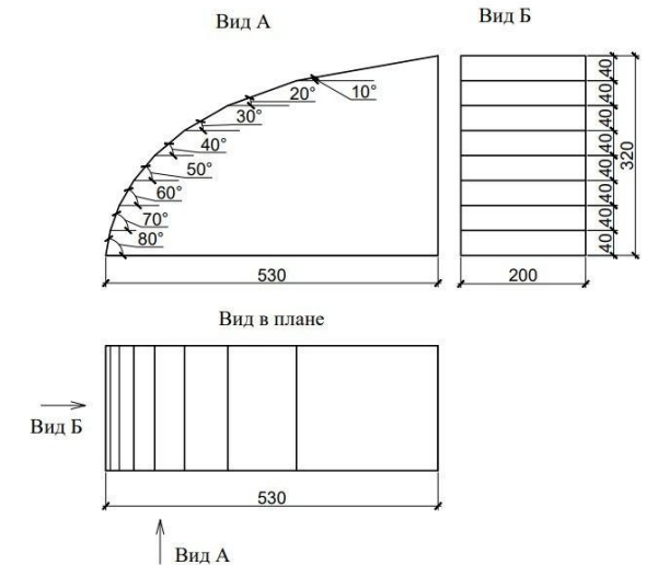
Эскизы экспериментальной установки
